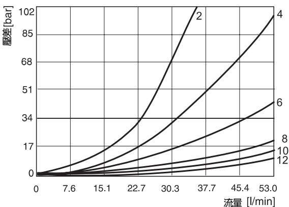
FM3, 單向閥流量
