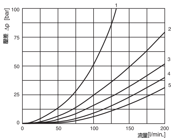
FM4，帶有標準針閥結構 針閥轉動1至5
