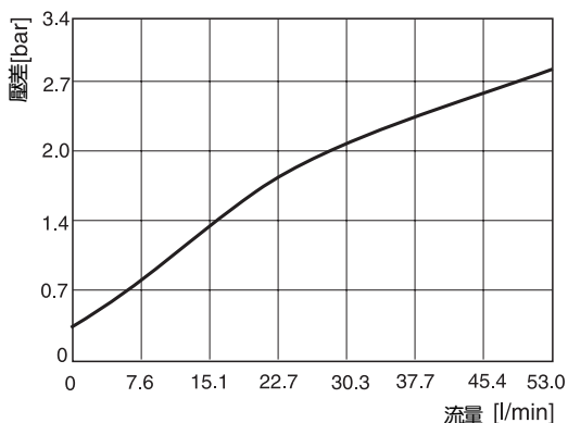
FM2, 標準錐形針閥結構
