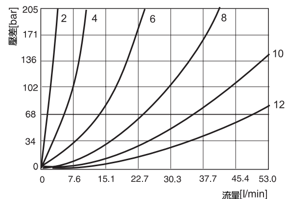
FM2G, 帶有平行溝槽的針閥結構
