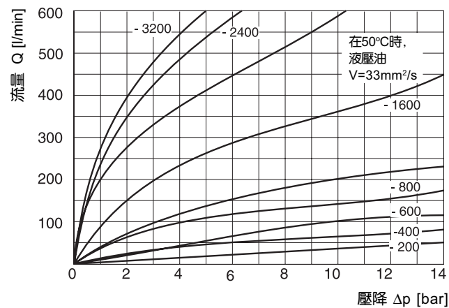
流量與針閥全開時的壓降
