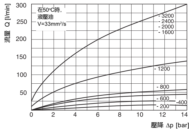
調節流量與針閥的壓降
