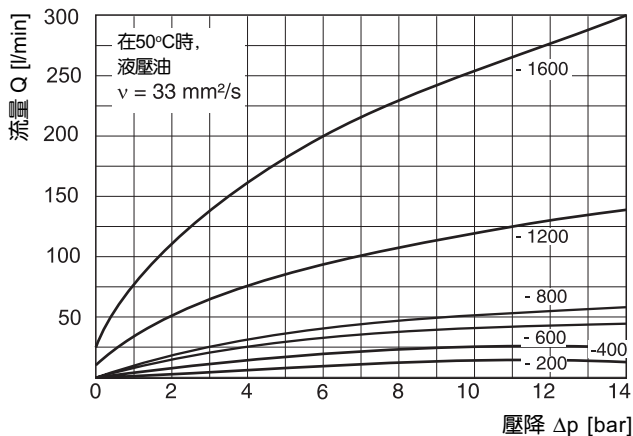
p/Q 特性曲綫
