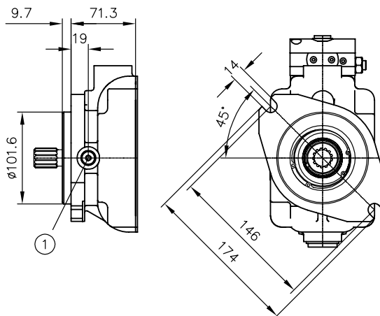
图片 23: 法兰结构形式 X
