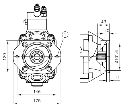
图片 49: 法兰结构形式 C024
