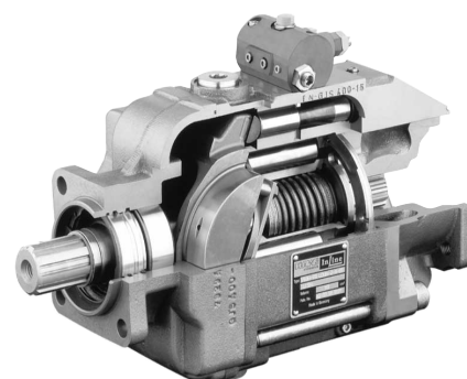
图片 1: V60N-110 型变量轴向柱塞泵
