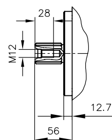
图片 44: 花键轴标记 S
