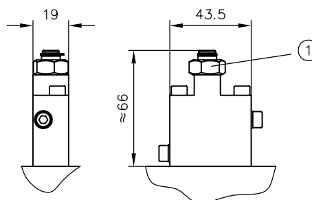
图片 65: 控制模块标记 /L
