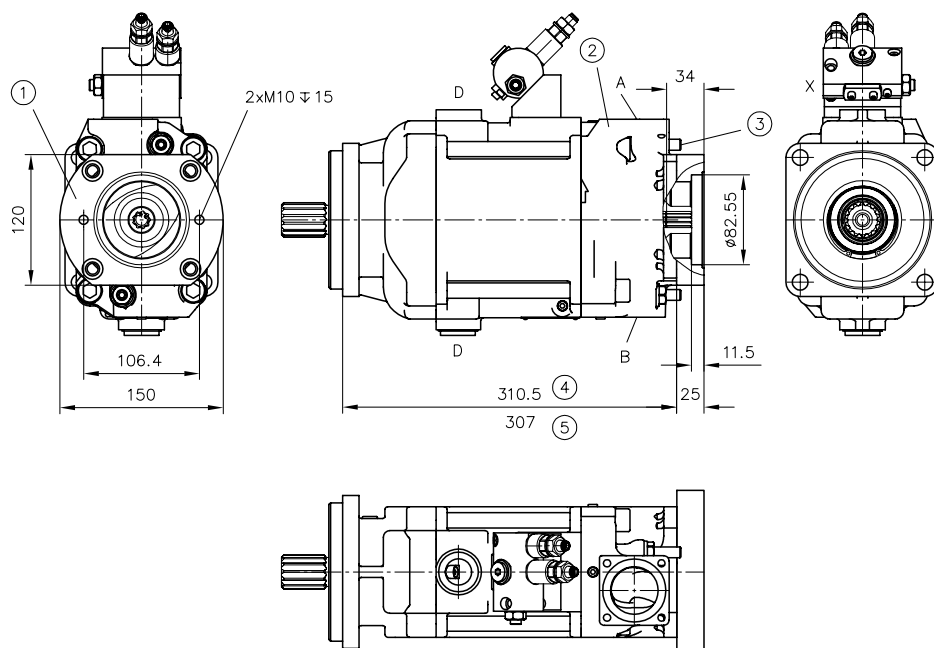
图片 35: 法兰结构形式 C 021、C 022 和 Y、F
