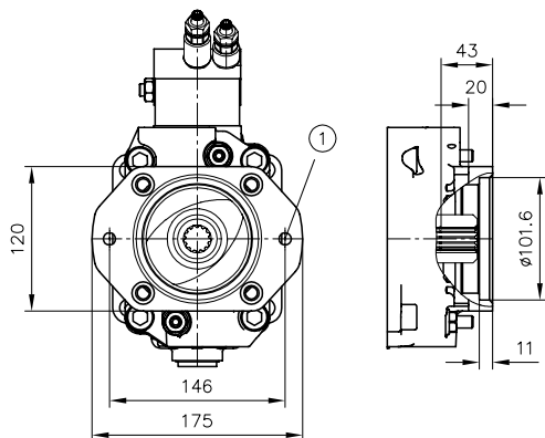
图片 36: 法兰结构形式 C024
