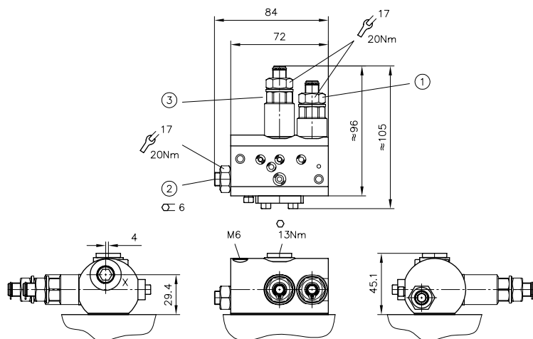
图片 62: 标记 LSNR、NR
