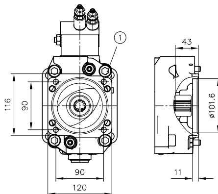
图片 37: 法兰结构形式 C025
