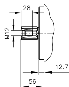
图片 15: 花键轴标记 S
