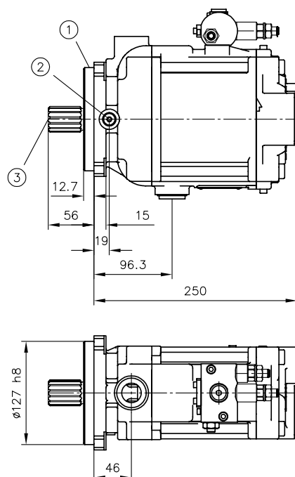
图片 14: 法兰结构形式 F
