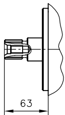
图片 32: 带法兰结构形式 Y 的花键轴 M
